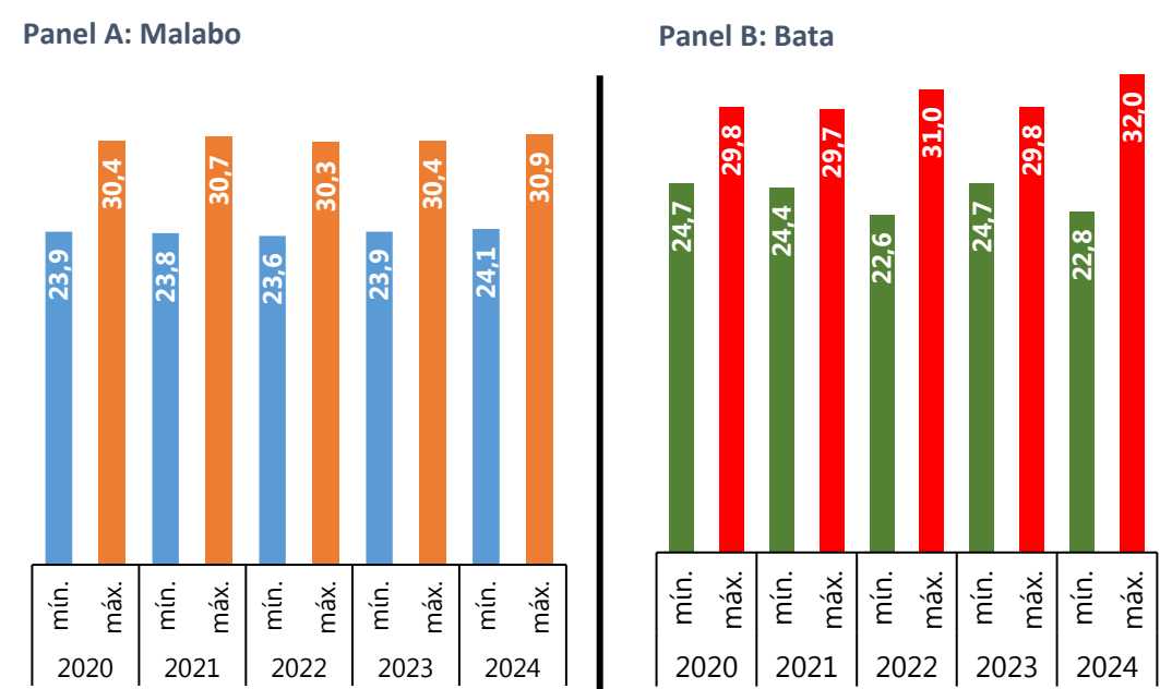
Gráfico 1: Evolución de Temperatura media anual en °C
