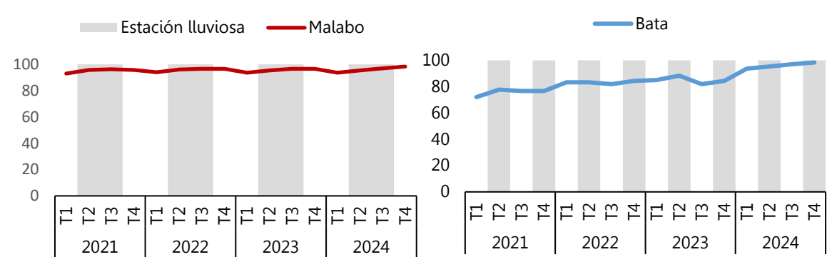
Gráfico 4: Humedad relativa media mensual (%)
