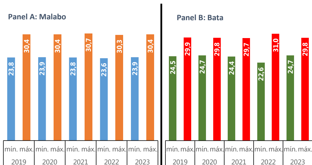
Gráfico 1: Evolución de Temperatura media anual en °C
