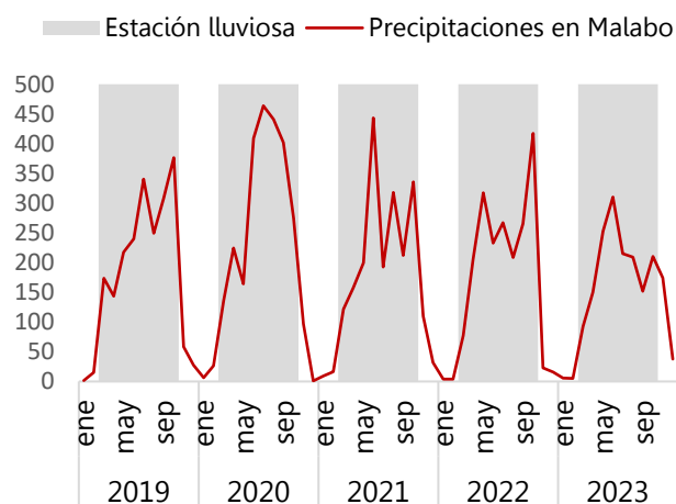
Gráfico 3: Volumen de precipitaciones (mm)
