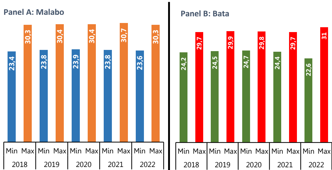
Gráfico 1: Evolución de Temperatura media anual en °C
