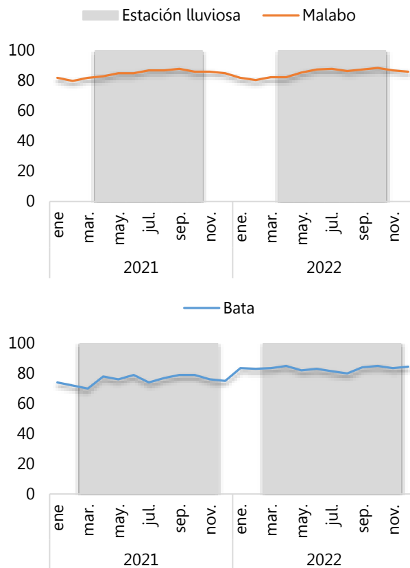
Gráfico 4: Humedad relativa media mensual (%)
