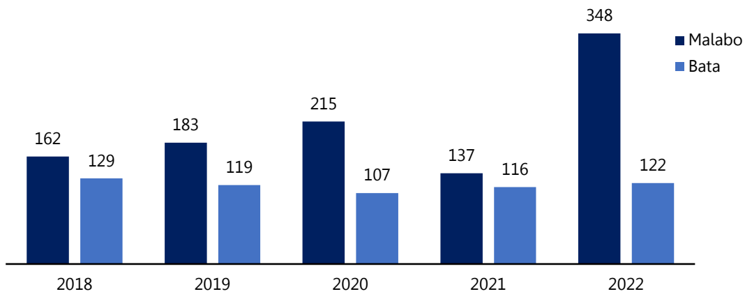
Gráfico 2: Evolución anual del número de horas con precipitaciones
